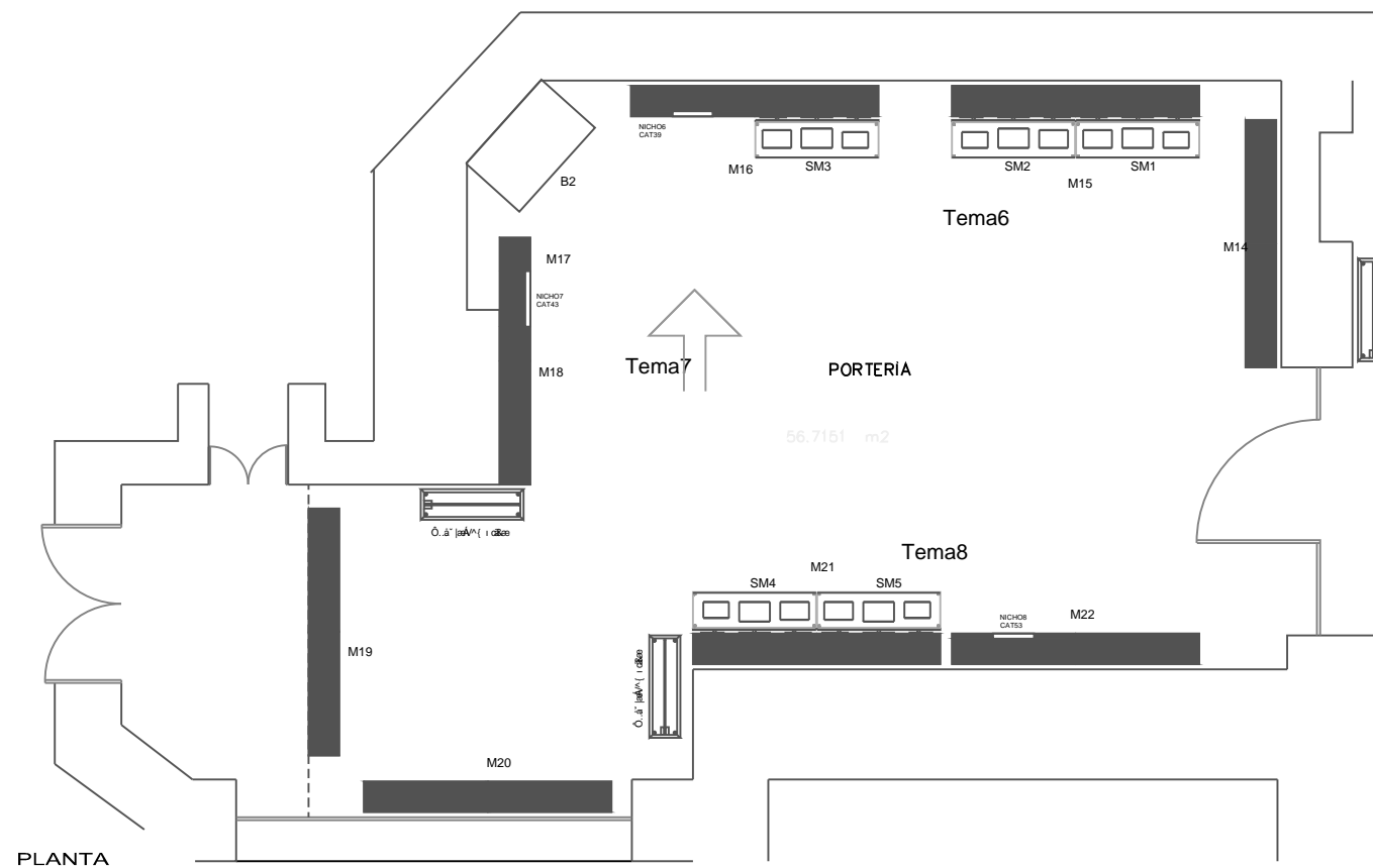
PLANTA
