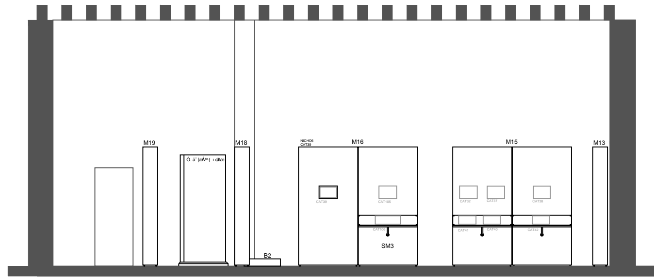
ALZADO
